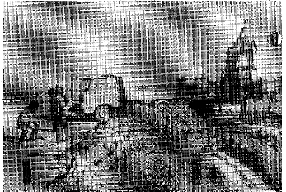
극동지구공병단 민간계약업체 직원들이 1983년 10월 오산 공군기지 현장에서 작업하고 있는 모습. 이들은 총670만불의 보수공사 중 그 일부분인 본 활주로의 연결되는 부활주로의 신축공사도 담당하였다. 이렇게 긴급을 요했던 공군이 발주한 공사는 상호간의 긴밀한 협조로 인하여 성공적으로 이루어질 수가 있었다.
