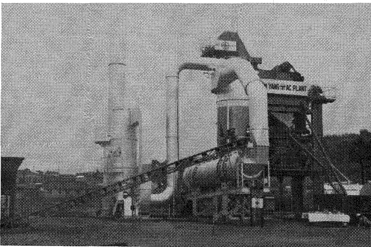
공사기간동안 범양에서 사용할 새아스팔트 뱉치공장
