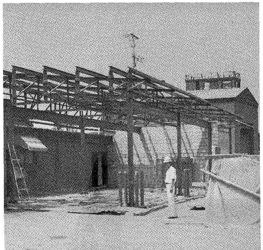
공사중인 미 육군 공수사령부의 대합실 건물
