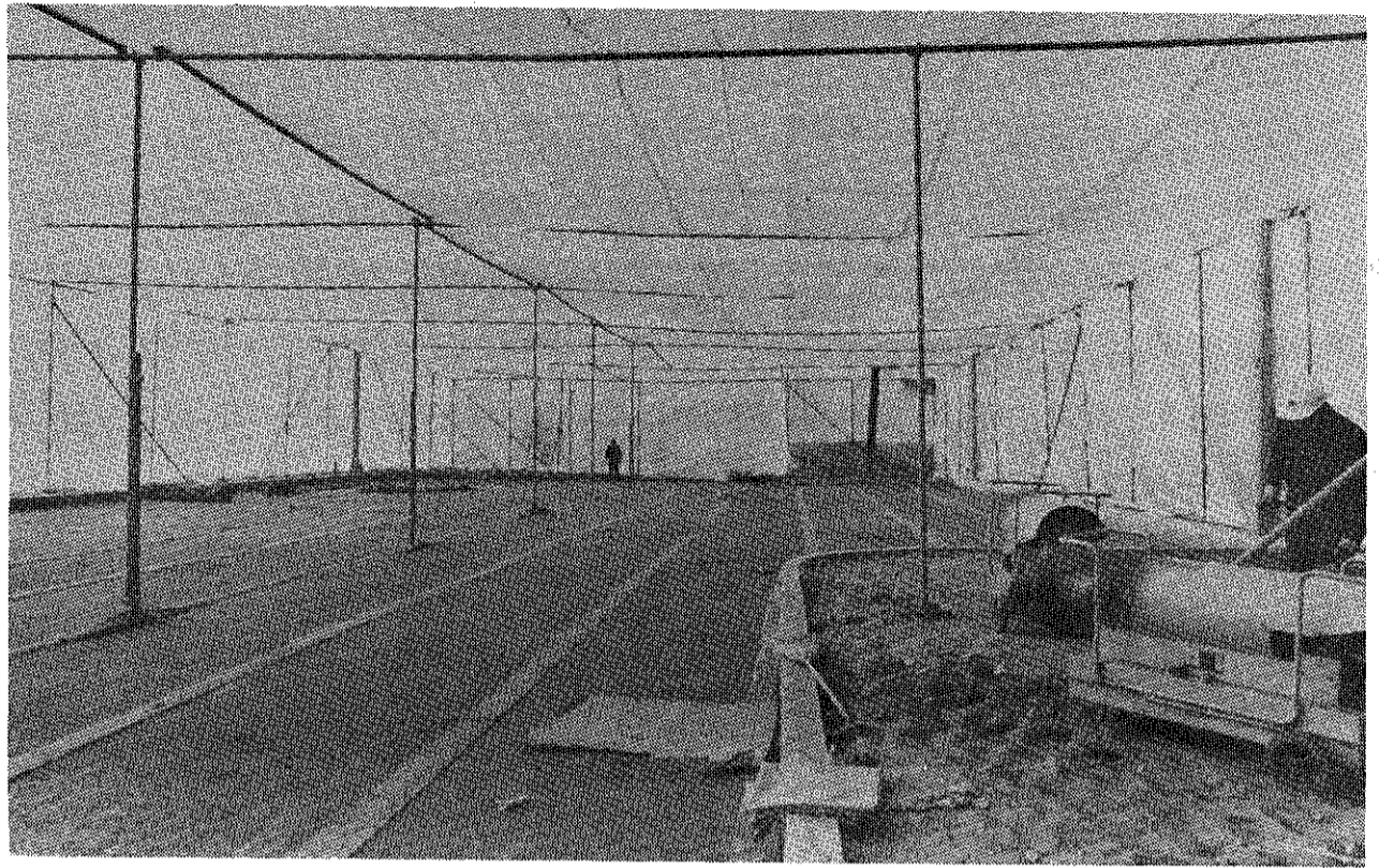
추운날씨에도 불구하고 진행되는 용산 청년회관 주차장을 건설하기 위하여 현장에 천막과 난로가 설치되었다.
