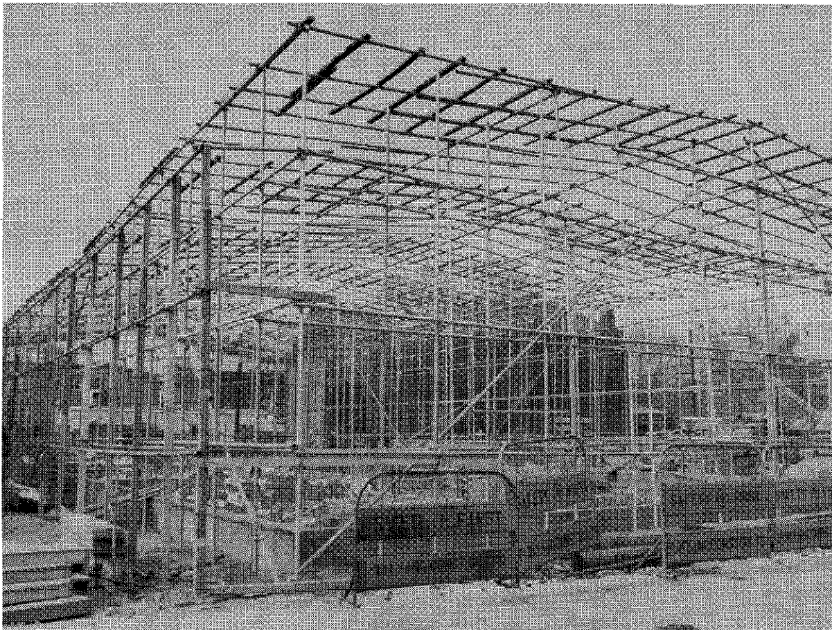
추운날씨에도 공사를 계속하기 위한 월동준비의 일환으로서 공사장에 천막을 씌울 준비를 하고 있다.
